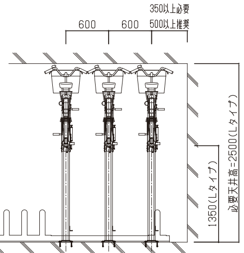
正面図 (ロータイプ)
