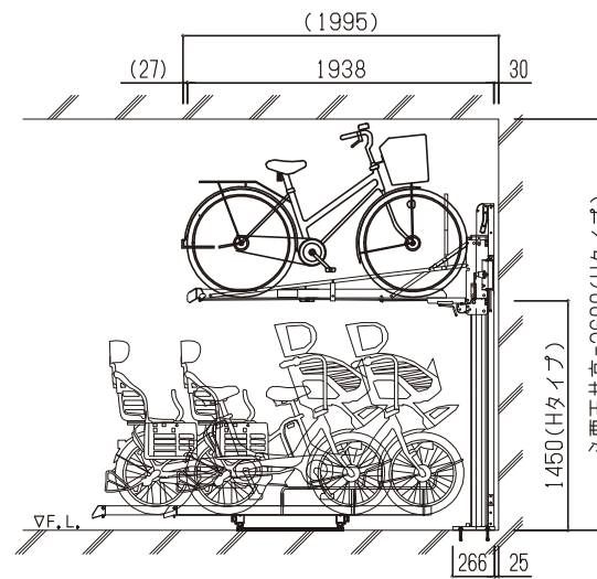
側面図 (ハイタイプ)
