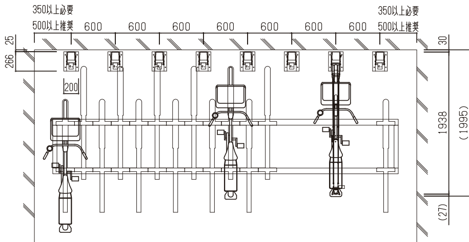
平面図 (ロータイプ)
