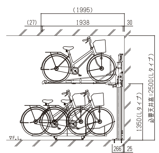
側面図 (ロータイプ)
