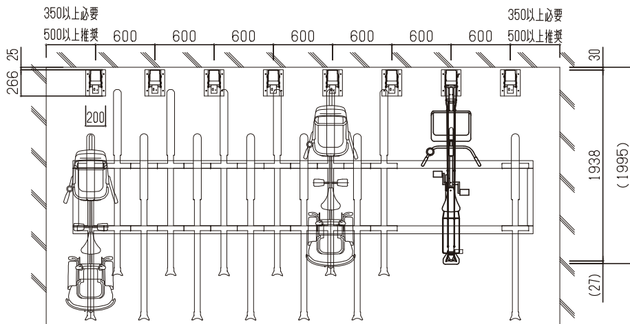
平面図 (ハイタイプ)
