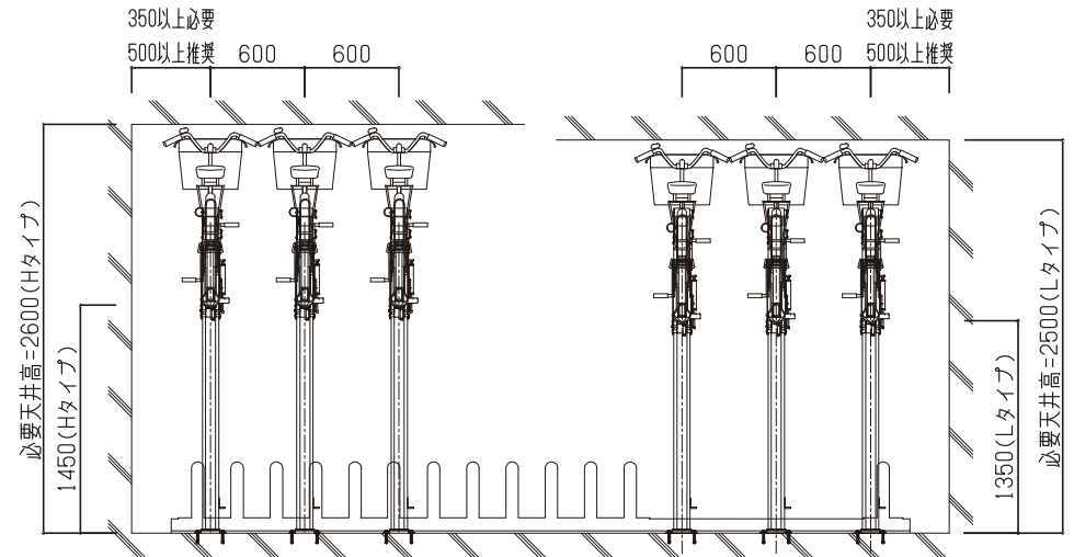
正面図 (ハイタイプ)
