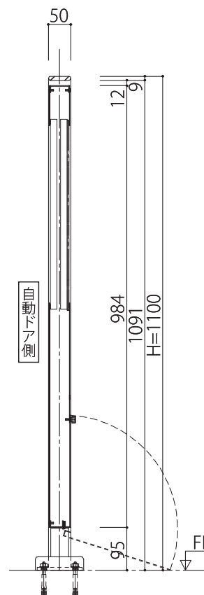
【断面図】
