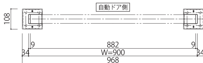
【平面図】
