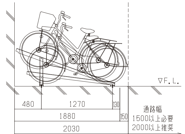
侧面图
