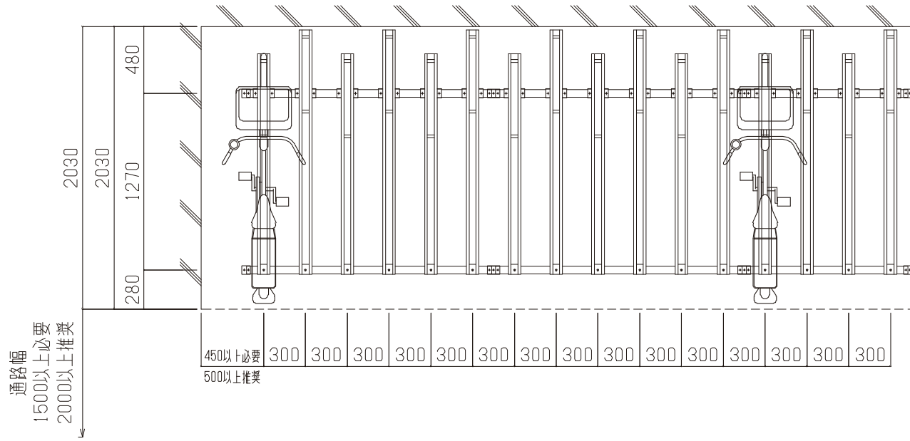
平面图
