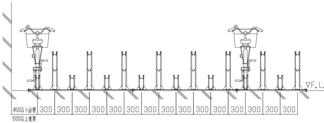
正面图
