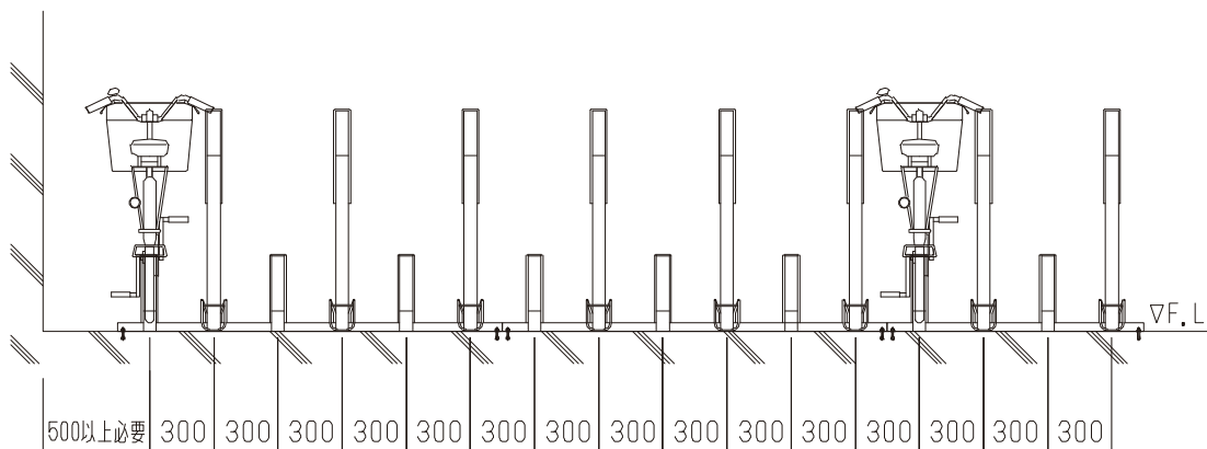
正面図
