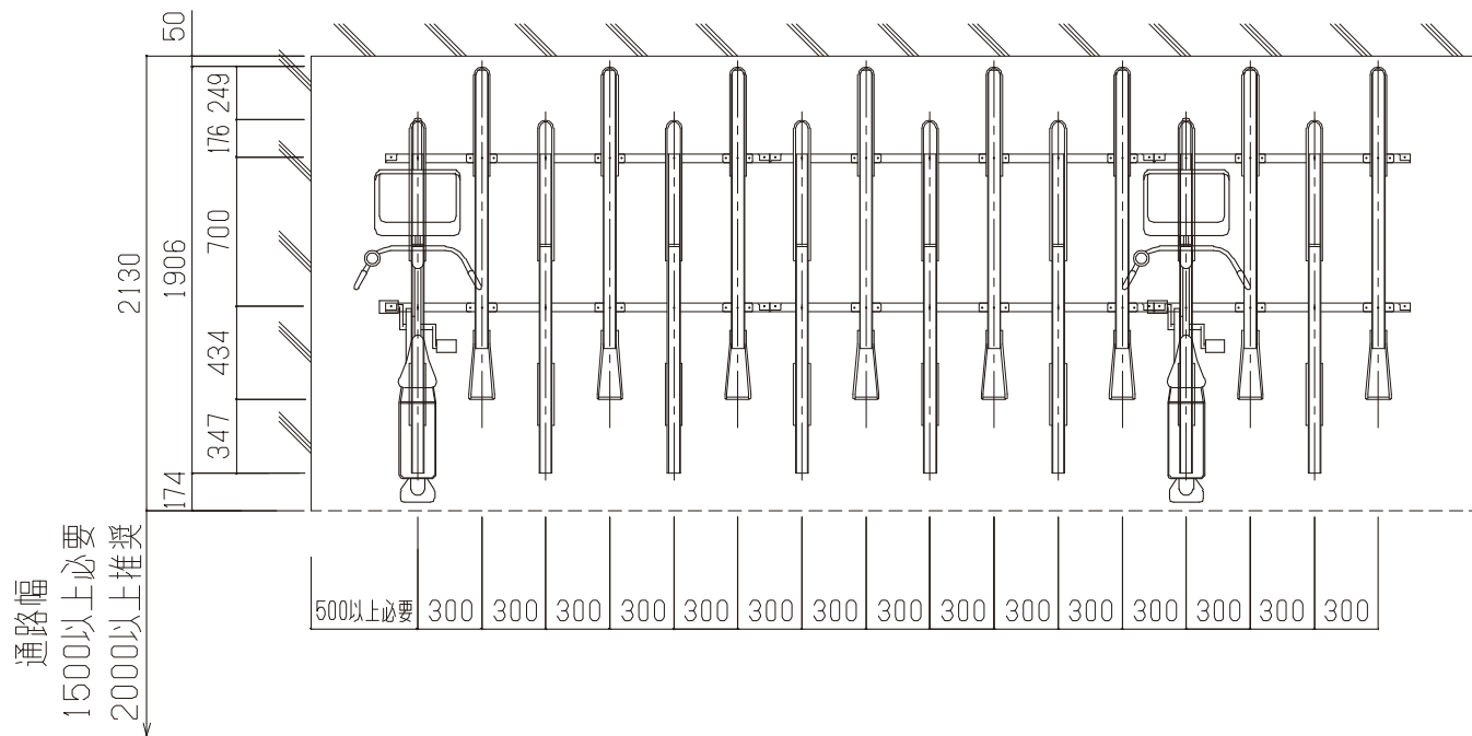
平面図
