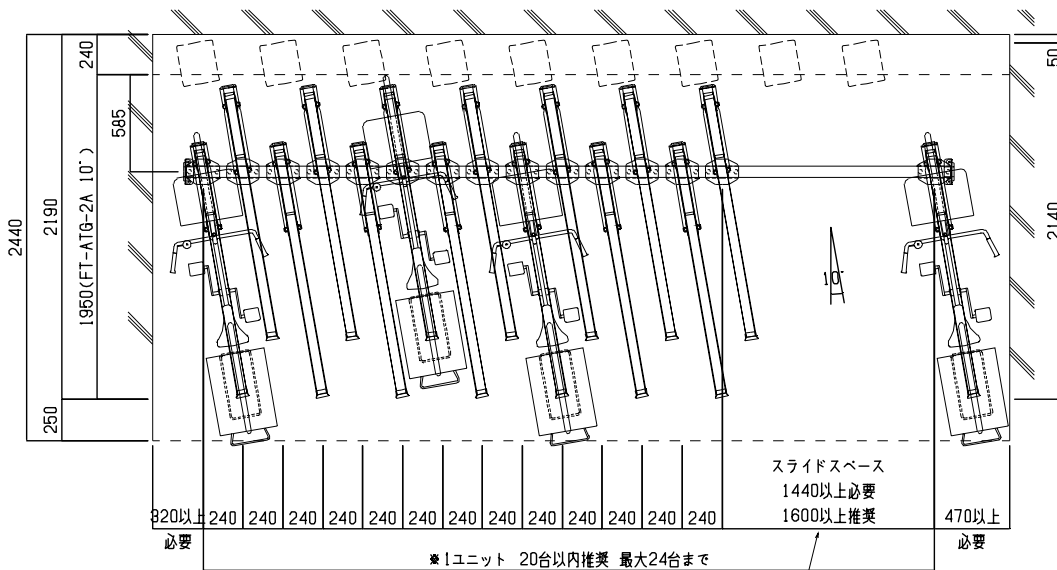
平面図（下段ラック）
