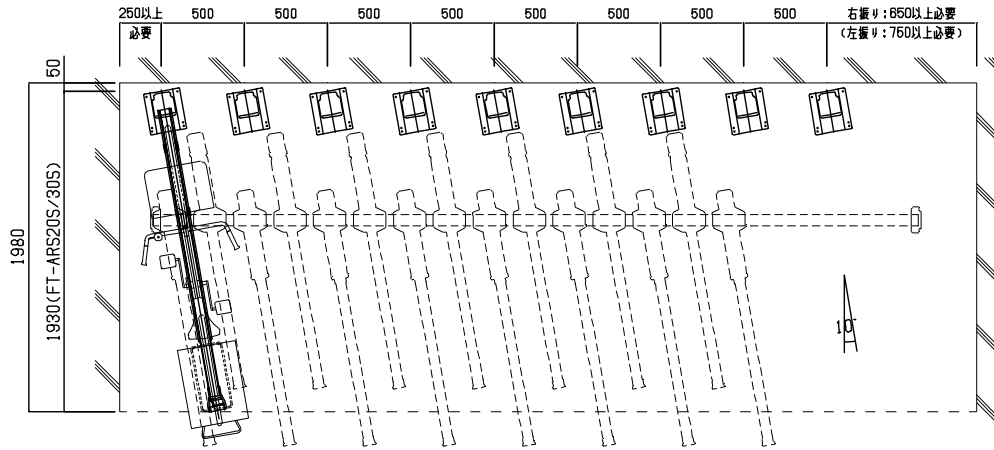
平面図（上段ラック）
