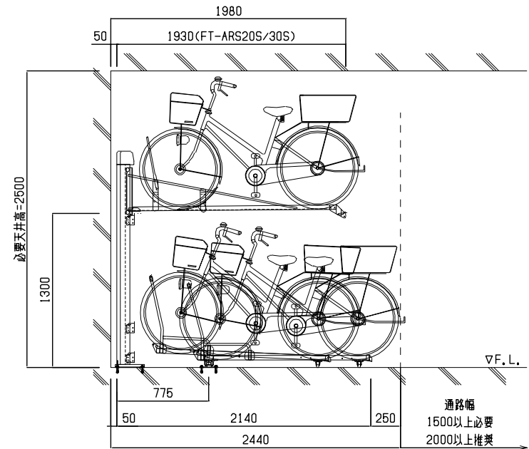
側面図
