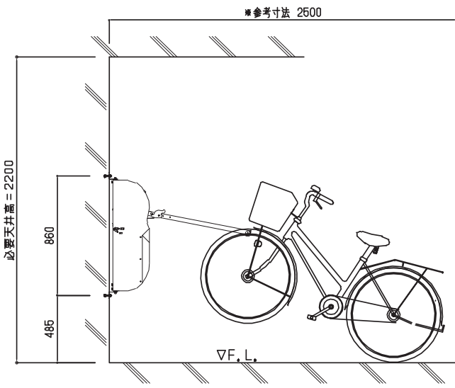
側面図 (収納前-H)
