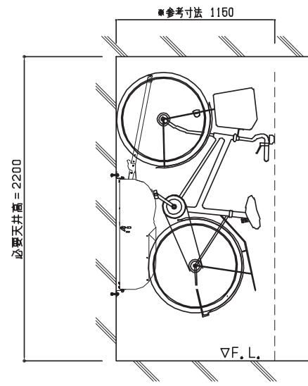
側面図 (収納後-H)
