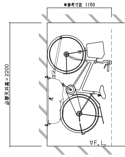
側面図 (収納後-L)
