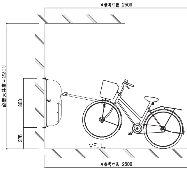
側面図 (収納前-H)
