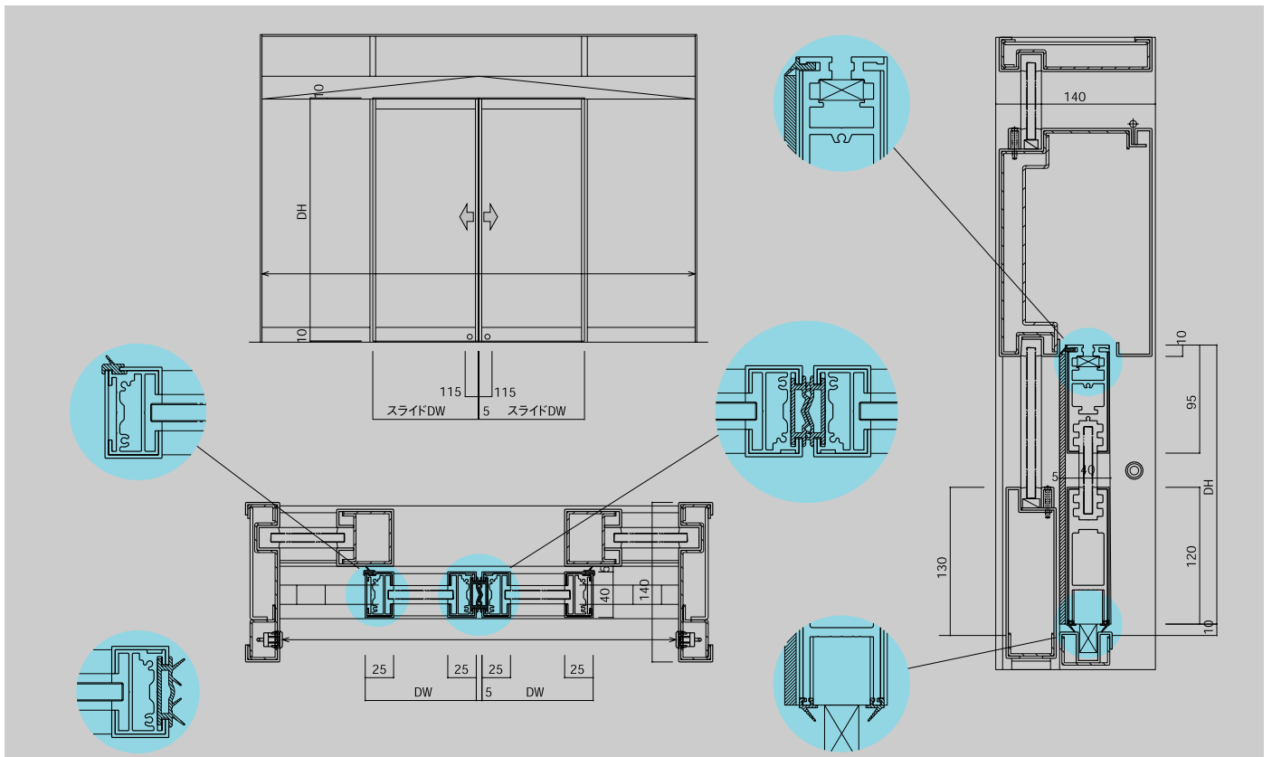
スリムタイトドア40 S/SL (ステンレス・スライド)
