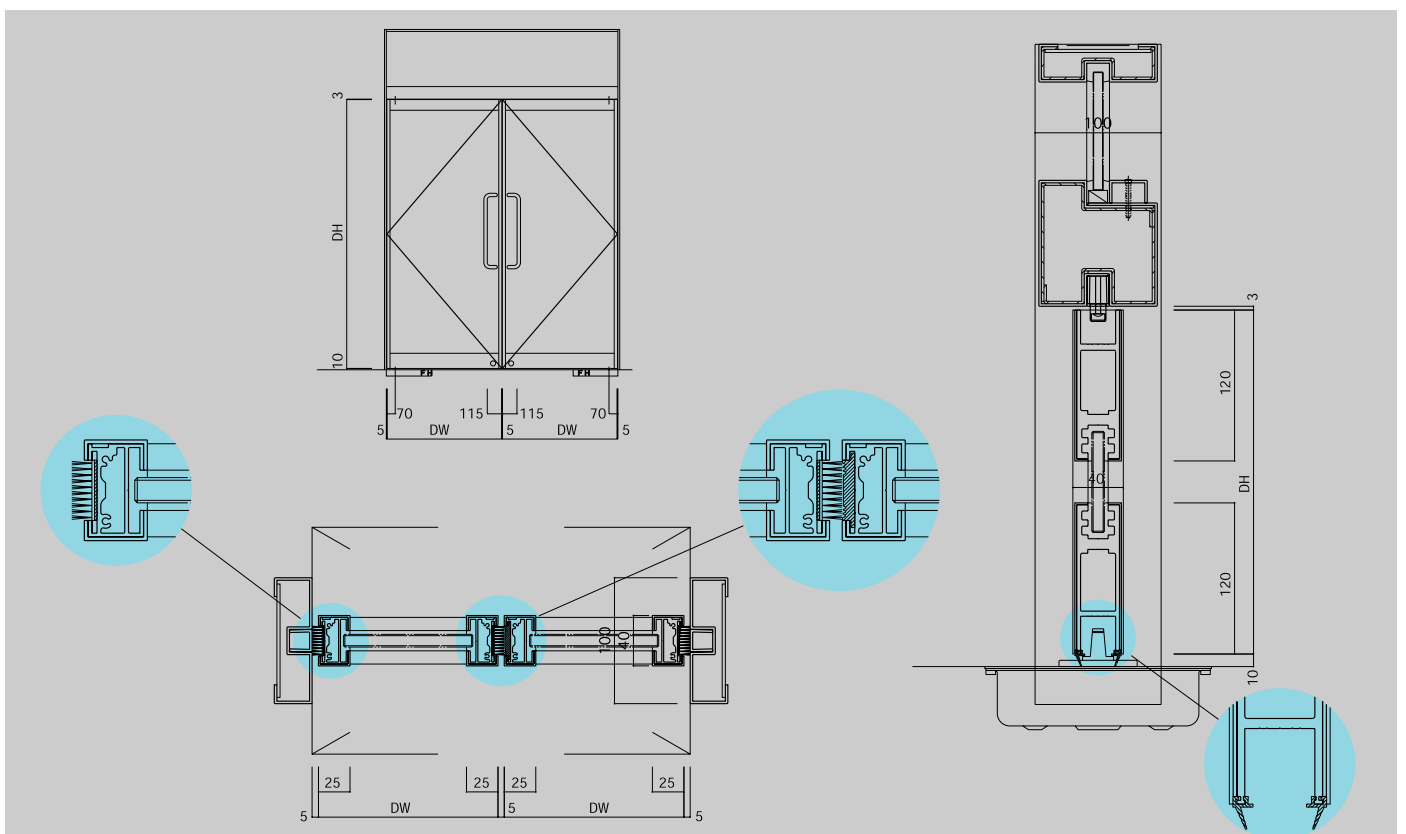
スリムタイトドア40 S/SW (ステンレス・スイング)
